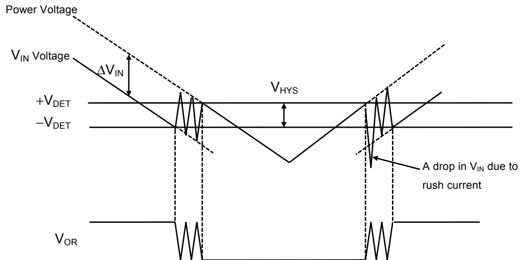
Figure 24 When \Delta V_{IN} > V_{HYS}
