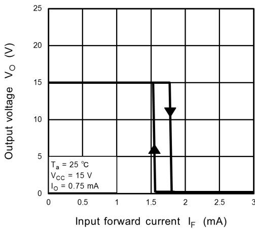
Fig. 12.2.9 V_O - I_F
